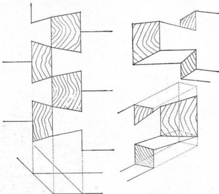
Fig. 7. Felul de îmbinare al bânelor la colțurile în unghi obtuz (Biserica din Zătrești).
