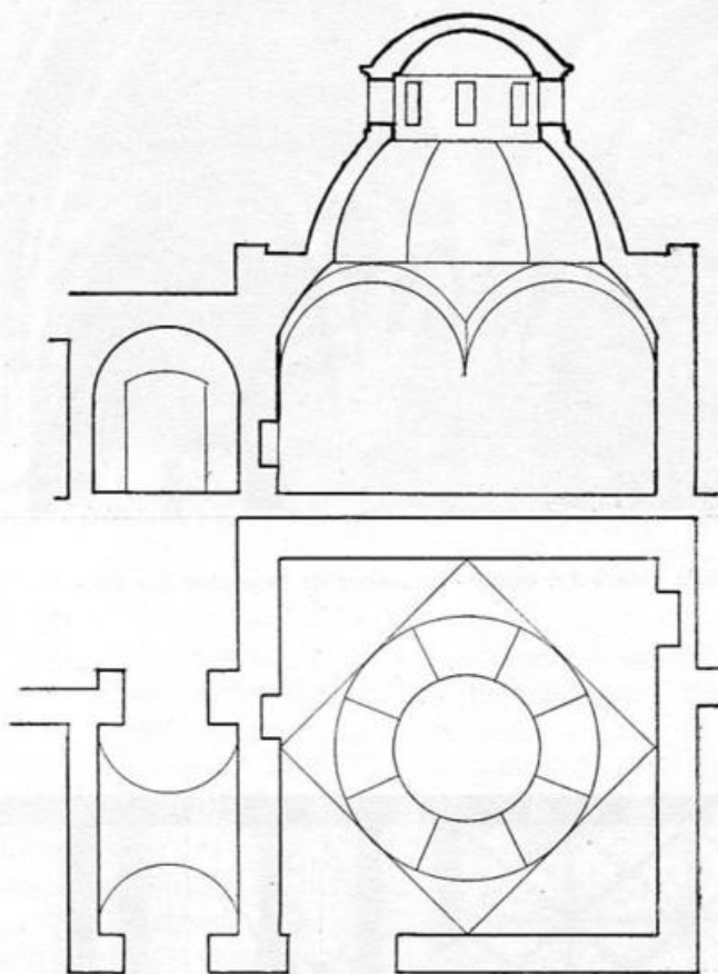
Fig. 340. Bucătăria de la mănăstirea Plumbuita lângă Bucureşti Plan şi secție.
