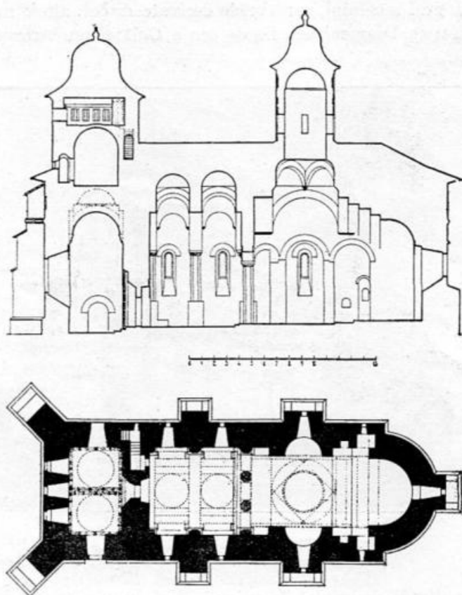
Fig. 294. Biserica mănăstirii Bărnova. Secție și plan.
