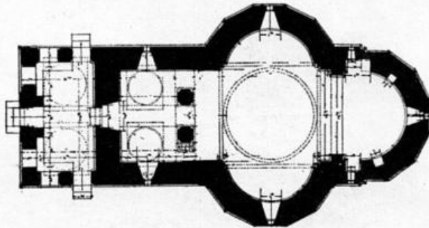
Fig. 112. Biserica mănăstirii Gura Motrului. Plan.
