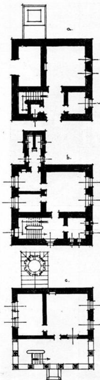
Fig. 360. Cula din Curtișoara jud. Gorj. Planuri : a. pivnița ; b. parterul ; c. etajul.
