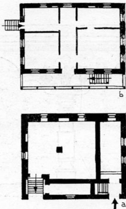
Fig. 356. Casa Dobrescu din Ploești : a. planul pivnițelor ; b. planul etajului.
