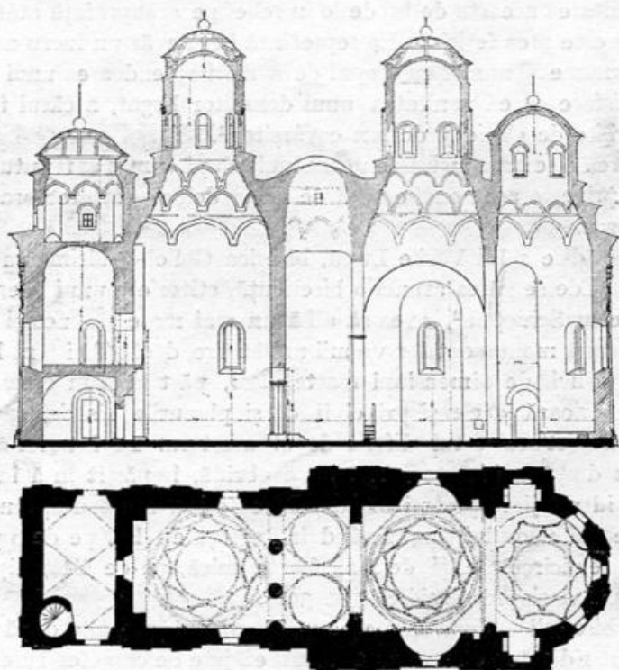
Fig. 302. Biserica Golia din Iași. Secție și plan. (După G. Balș).
