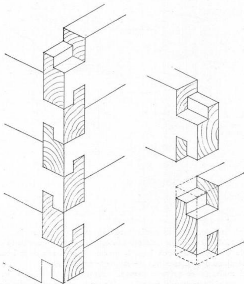
Fig. 6. Felul de imbinare al bânelor la colțurile în unghi drept (Biserica din Zătreni).
